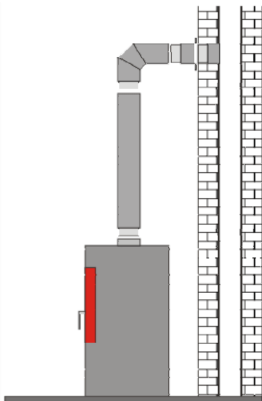
Zapojení kouřovodu „po vodě“
