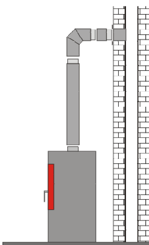
Zapojení kouřovodu „po kouři“
